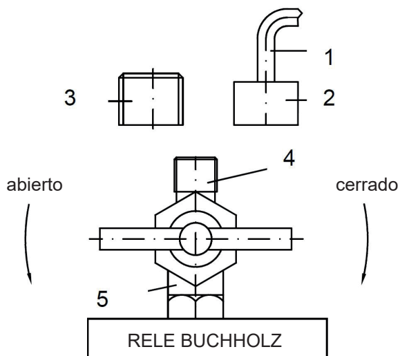
Figura 3 - Control en el relé Buchholz
