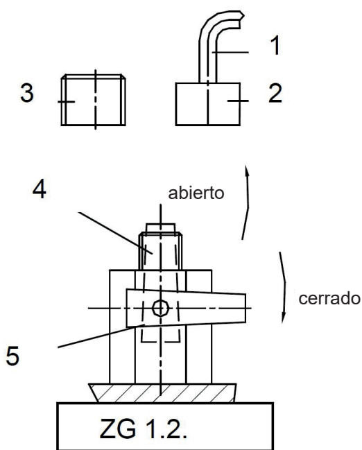
Figura 4 - Control mediante el ZG 1.2.
